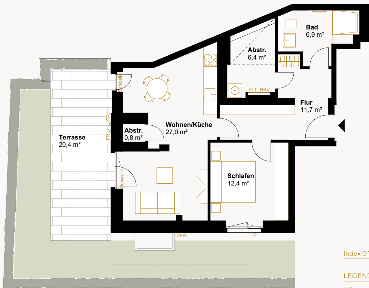
GESCHOSSPLAN
