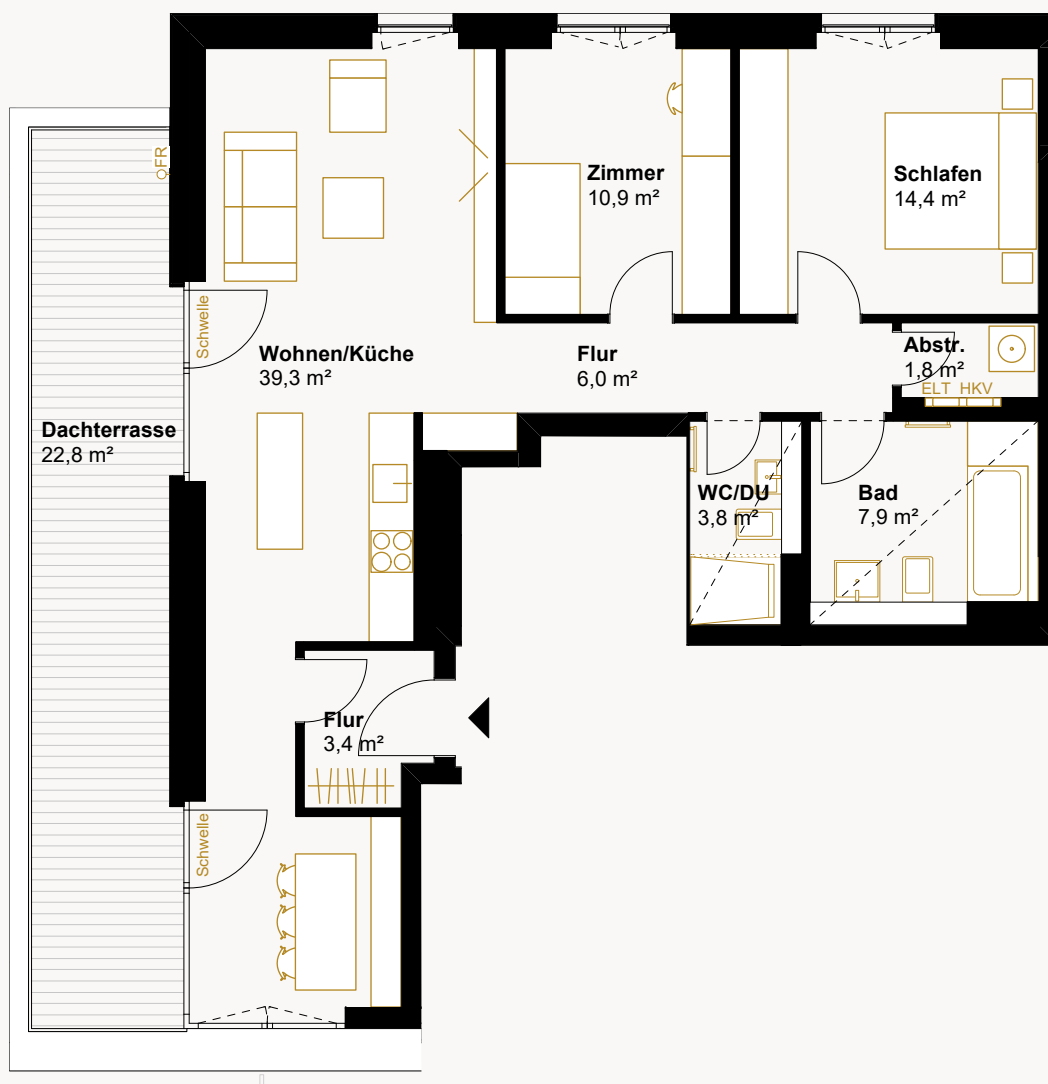
GESCHOSSPLAN
